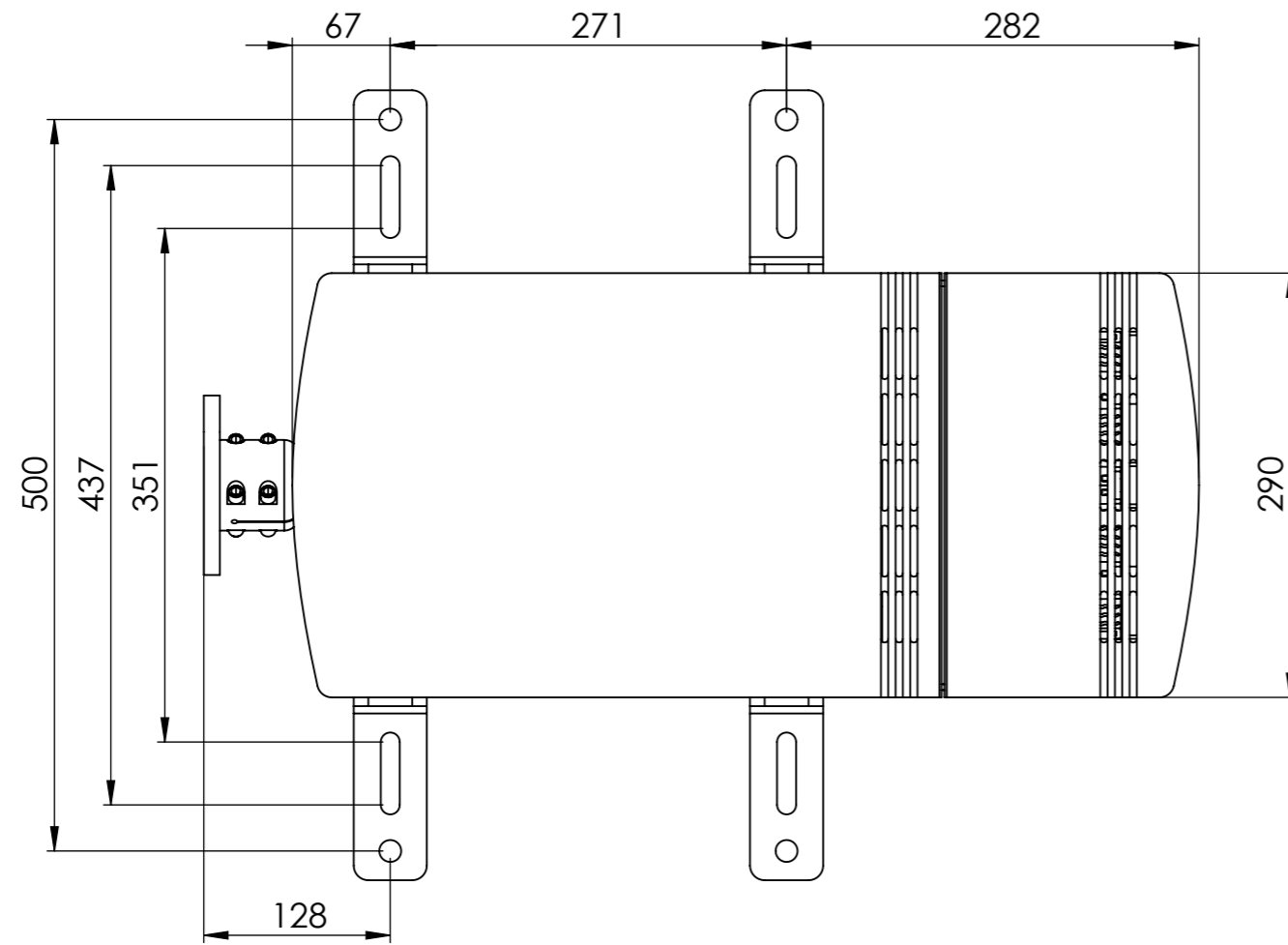
Aanzicht Zij
